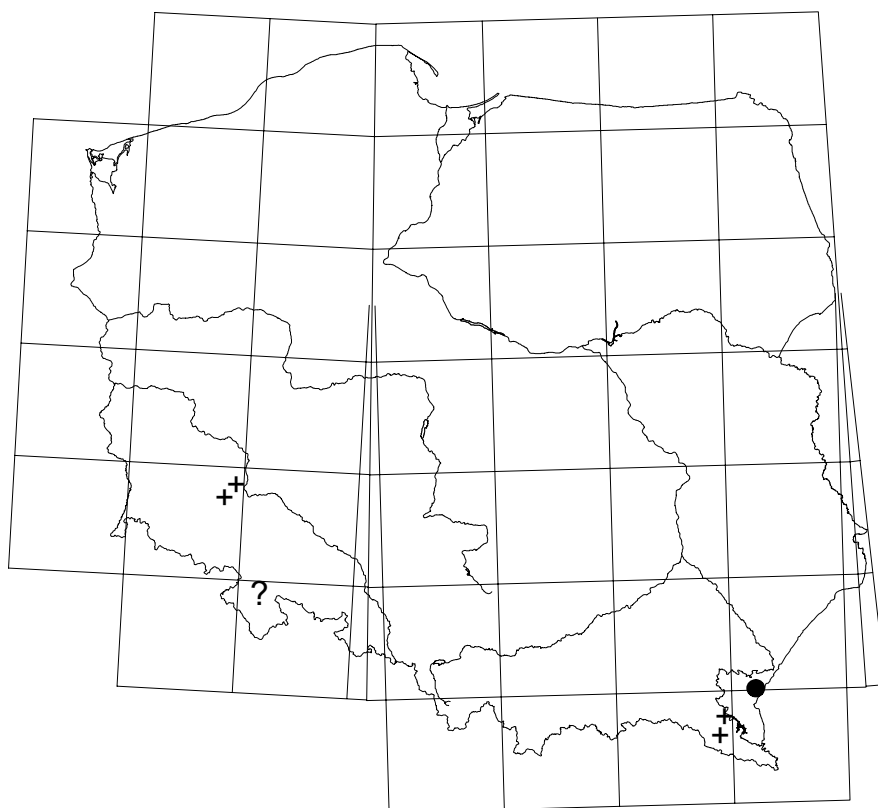
Ryc. Stanowiska Encarta amethystina (HBN.) w Polsce: + – stanowiska historyczne, ● – stanowisko po roku 2000, ? – stanowisko wątpliwe
